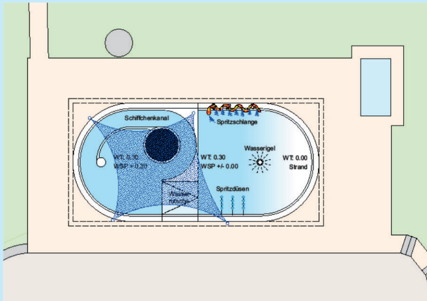
Grundriss des neuen Kinderplanschbeckens
